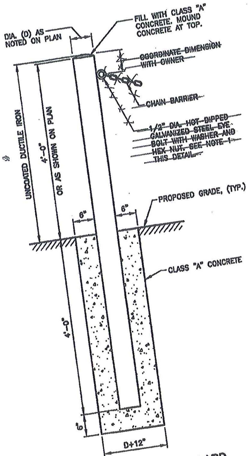
DUCTILE IRON (D.I.) BOLLARD N.T.S.
